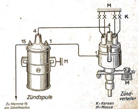
Bild 5 Zündspule und Zündverteiler
