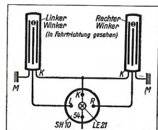
Bild 6 Winker mit Federkontakt für Anzeigelaterne
