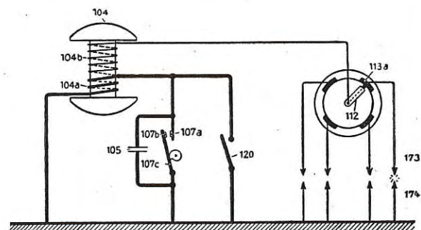
Bild 10 Grundsätzliche Schaltung eines Magnetzünders
