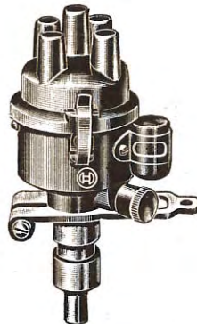
Bild 3 Zündverteiler VE 4
