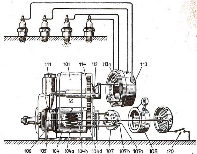
Bild 9 Magnetzündler mit umlaufendem Anker
