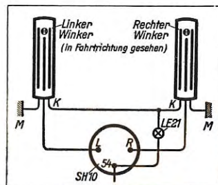
Bild 5 Winker mit Federkontakt für Anzeigelaterne
