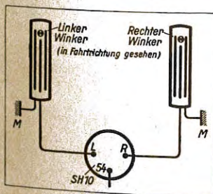
Bild 4 Winker ohne Federkontakt für Anzeigelaterne
