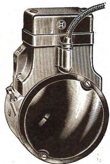
Bild 7 Schwung-Lichtbatteriezünder F 1 LK
