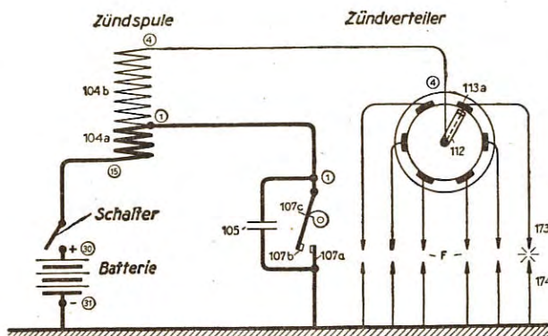
Bild 6 Grundsätzliche Schaltung der Batteriezündung
